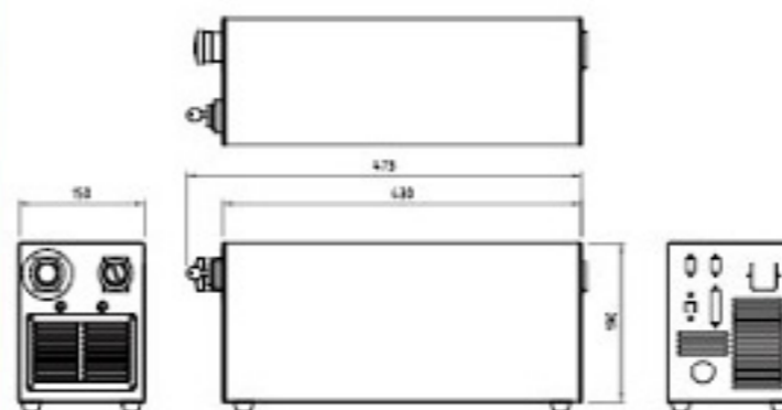
V30 控制箱
